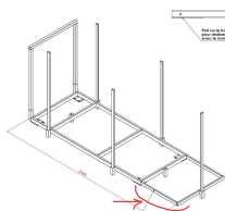
Rallonge Réf CHTAB-RA244
